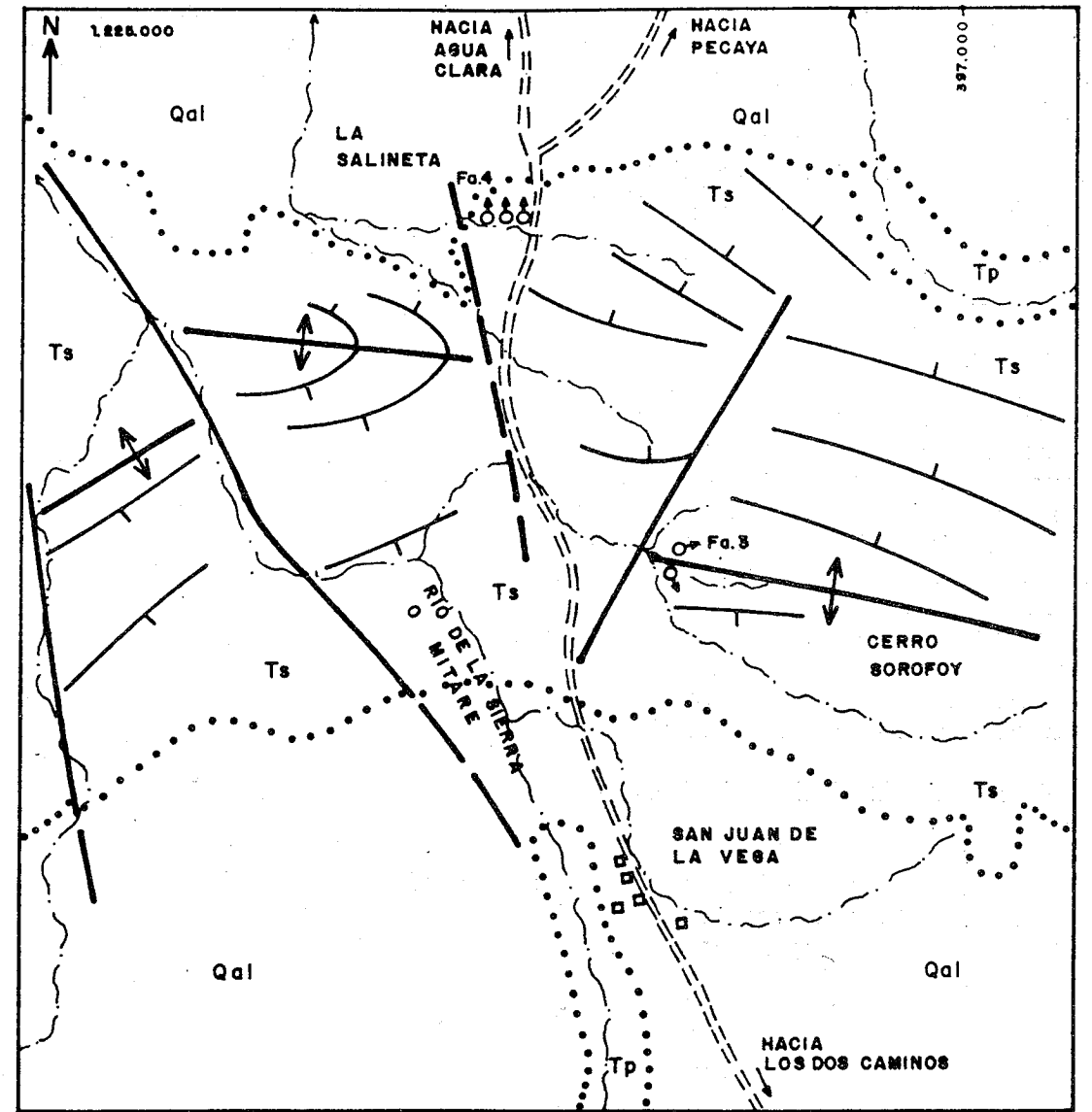
FIG. 38. MAPA GEOLOGICO Y DE UBICACION DE LAS FUENTES TERMALES DE SALINETA Y SOROFOY, PECAYA, EDO. FALCON (Fa. 3 y 4)
