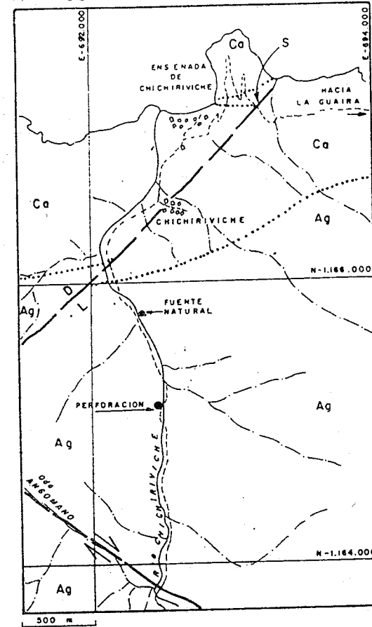
A MAPA GEOLOGICO Y DE UBICACION DE LAS MANIFESTACIONES GEOTERMICAS DEL AREA DE CHICHIRIVICHE, D.F.
