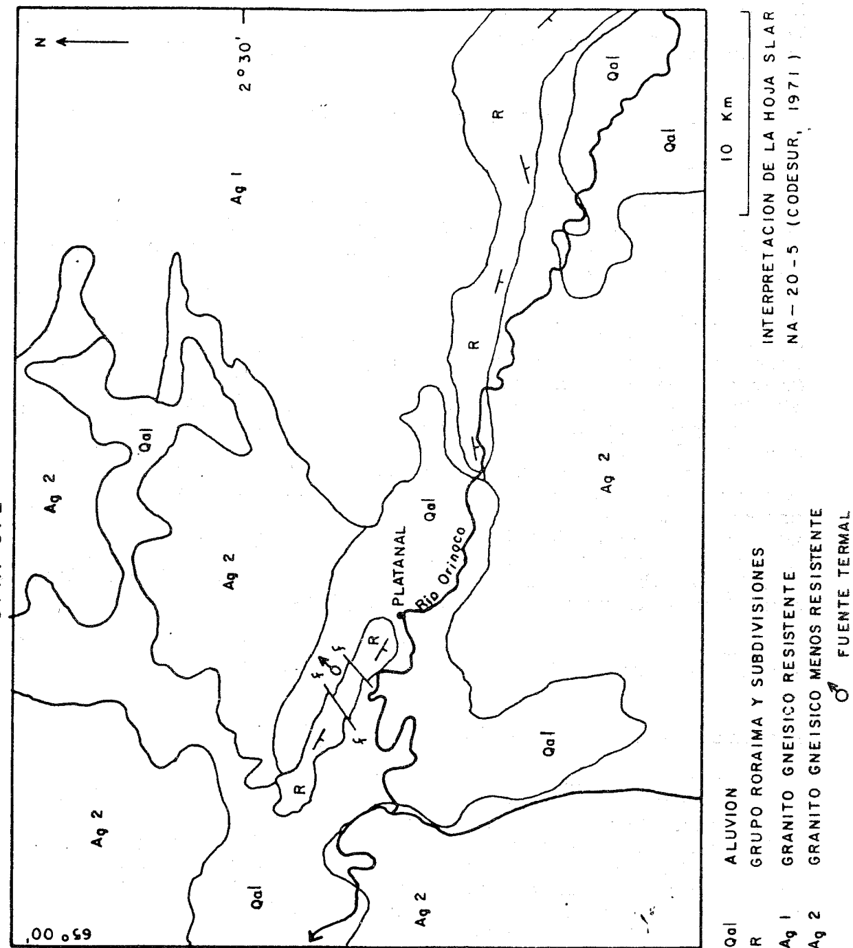
MAPA GEOLOGICO DEL AREA DE PLATANAL, T.F. AMAZONAS Y UBICACION DE LA FUENTE TERMAL DE YOPRI-UPE
