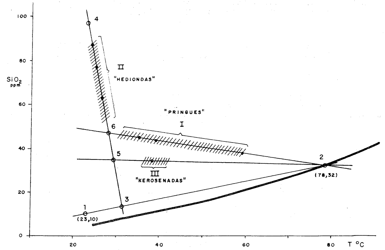
FIG. 133 MODELO DE MULTIPLES MEZCLAS PARA LAS AGUAS TERMALES DE AGUAS CALIENTES, UREÑA, TACHIRA. (GRAFICOS SIMILARES PUEDEN CONSTRUIRSE CON EL EJE Y= T.S.D, CI)
