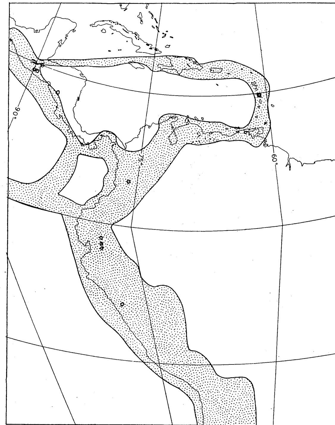
Zona punteada: Zona con emisiones de CO 2 Círculos: Emisiones fuertes de CO 2 estudiadas por BARNES et al., 1978
