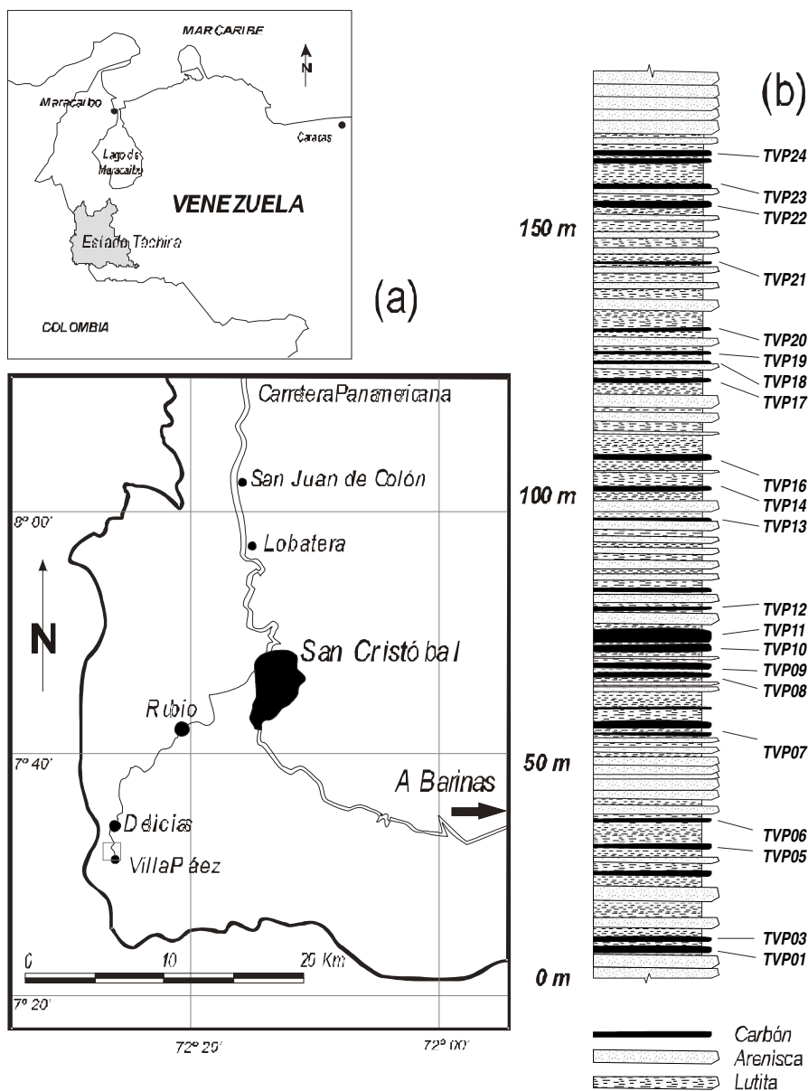
Figura 1. Ubicación de la zona de estudio (a). Columna estratigráfica de la Formación Los Cuervos en la región de estudio, indicando la nomenclatura de las muestras colectadas (b).
