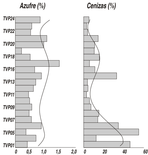
Figura 2. Variación vertical en la concentración de azufre y cenizas en los carbones analizados, en función de su posición en la columna
