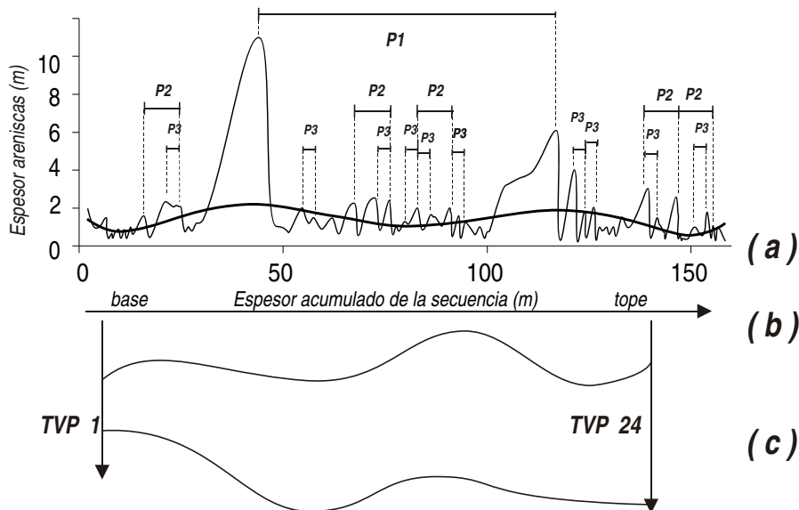
Figura 5. Patrón cíclico en la Formación Los Cuervos. (a) Patrón de variación en el espesor de las areniscas en la unidad estudiada. Se aprecia un gran ciclo de período aproximado 70-75 m (P1), un segundo ciclo de mayor frecuencia pero menor intensidad, con período aproximado 11 m (P2), y un ciclo menor, de período 5 m (P3).
