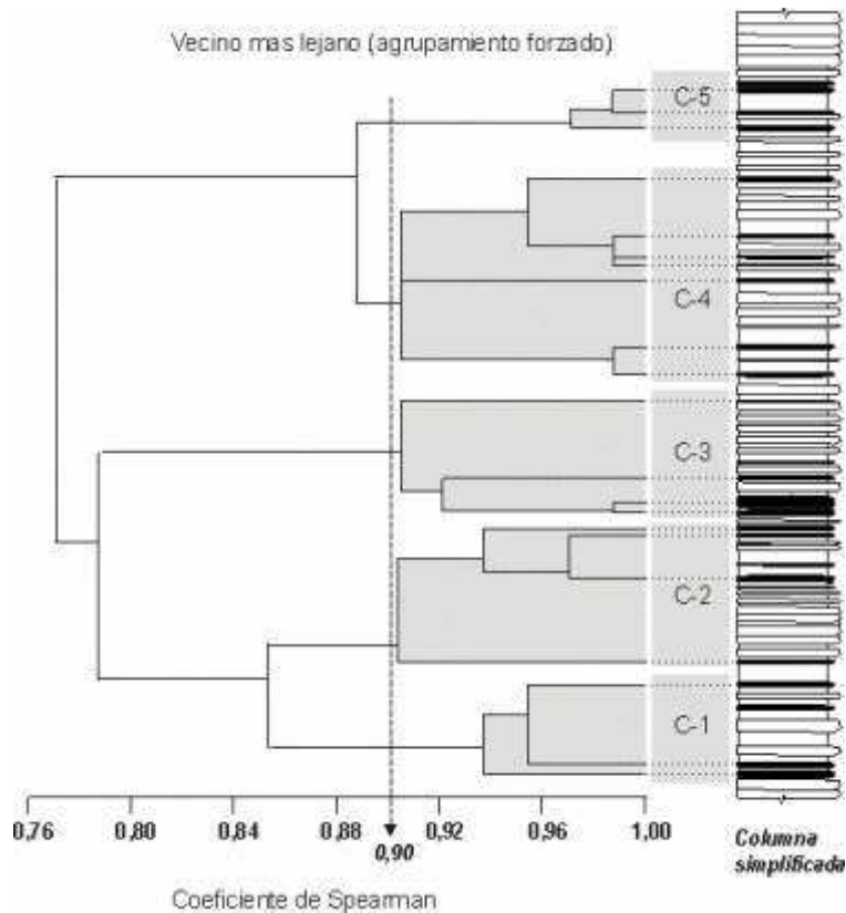
Figura 3. Análisis de agrupamiento forzado (“constrained clustering”) sobre los carbones estudiados, utilizando como variables los análisis inmediatos, elementales, azufre total y espesor de los mantos.
