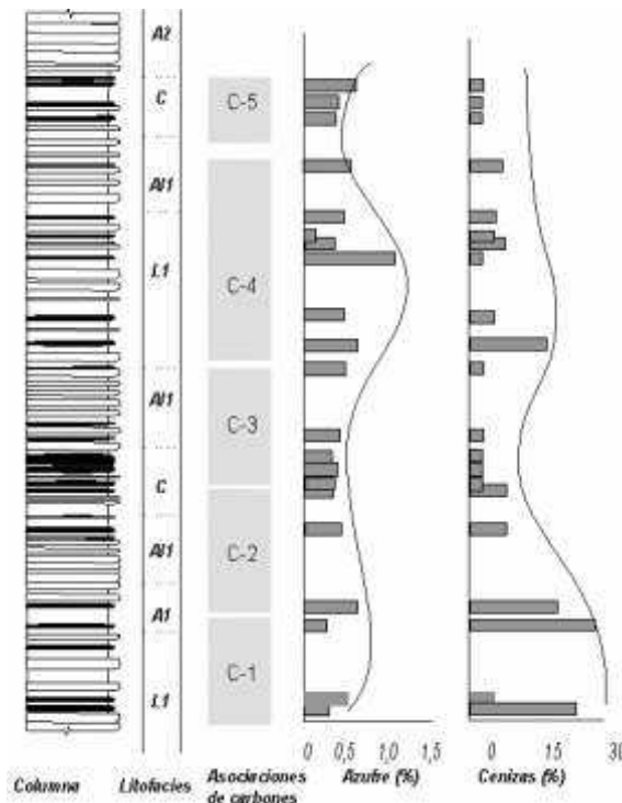
Figura 4. Correlación entre las litofacies sedimentarias y la variación vertical de azufre y cenizas (curvas de ajuste polinomial de grado 6) en los carbones de la Formación Los Cuervos en Villa Páez.
