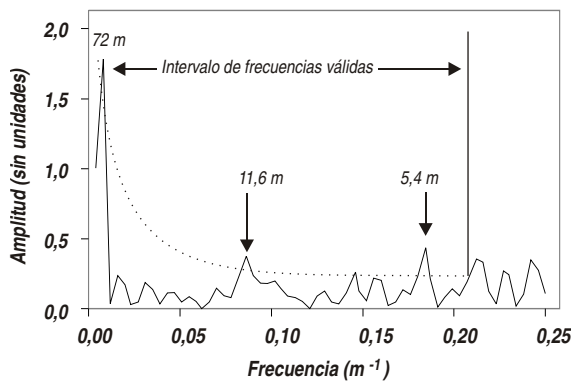
Figura 6. Análisis espectral de los valores de espesor de las areniscas, mediante Transformadas de Fourier (FFT).
