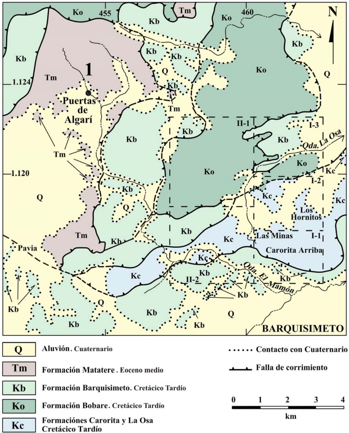
Figura 1b. Mapa geológico generalizado del norte de Barquisimeto, simplificado con modificaciones a partir de Bellizzia & Rodríguez (1967). El recuadro segmentado ubica a la Fig. 2. Los recuadros con siglas I-1 a II-2 correspondientes a las zonas de trabajo de las asignaturas Geología de Campo I y II de 1967. El número 1 señala una localidad fosilífera descrita en el texto.
