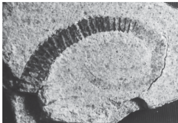
Figura 6a. Amonite del género Idiohamites de la Formación Carorita. Ancho de la fotografía 6 cm. Tomado de Seitz et al. (1968), también reproducido en Macsotay et al. (1987: 39).
