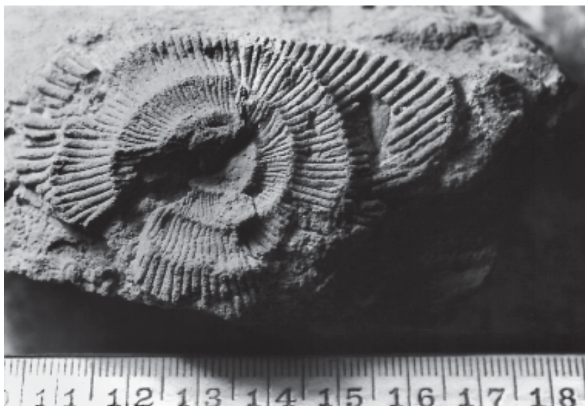
Figura 3. Molde de un amonite procedente de un olistolito de la Formación Matatere. Tomado de Urbani et al. (1968). Ha sido identificado en forma diferente por dos autores: 1) Nebroditas sp. del Jurásico Tardío por el Dr. Otto Renz, com. pers. 1986. 2) Prohysteroceeras sp. del Cretácico Temprano por Macsotay et al. (1987).
