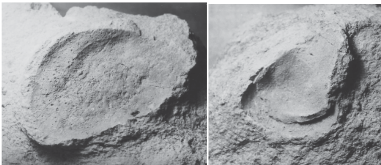
Figura 4. Moldes de Ostrea sp. de la Formación Bobare. Ancho de las fotografías 12 cm. Tomado de Urbani et al. (1968), fotografías e identificación por O. Macsotay en 1967.
