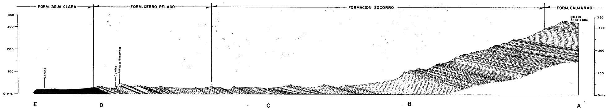
CORTE GEOLOGICO DE LA SECCION MEDIDA EN EL SALADILLO EDO. FALCON
