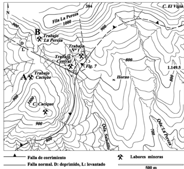
Figura 6. Mapa geológico-topográfico de la zona minera de San Jacinto. Simplificado a partir de LÓPEZ & BRINEMAN (1943). El recuadro ubica a la Fig. 7 y las letras A y B localizan secciones geológicas presentadas en la Fig. 14.
