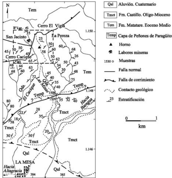
Figura 4. Mapa geológico de la zona de La Mesa - San Jacinto. Simplificado a partir de la hoja topográfica 6147-II-SE y la geología según WHEELER (1958), LÓPEZ & BRINEMAN (1943) y principalmente GODDARD & CASTILLO (1970). El recuadro ubica a la Fig. 6.
