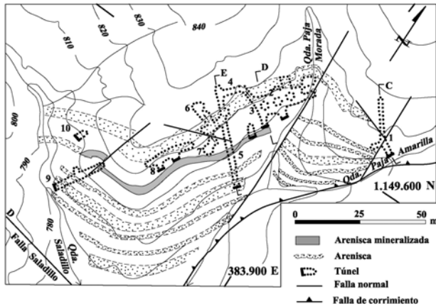
Figura 7. Mapa de los trabajos mineros de San Jacinto. La toponimia de las obras subterráneas según LÓPEZ & BRINEMAN (1943) es como sigue: 1: Trabajo No. 1, 2: Rabaje A, 3: "Winze", 4: Rebaje Norte, 5: Traviesa, 6: Rebaje Sur, 7: Realce Sur, 8: Trabajo No. 5, 9: Saladillo, 10: Trabajo No. 4. La geología y topografía ha sido simplificada a partir de GODDARD & CASTILLO (1970) y LÓPEZ & BRINEMAN (1943). Las letras C, D y E ubican secciones de la Fig. 14.
