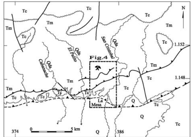
Figura 2. Mapa geológico de la región noreste de Carora. Modificado y simplificado a partir de WHEELER (1958). El recuadro ubica a la Fig. 4.
