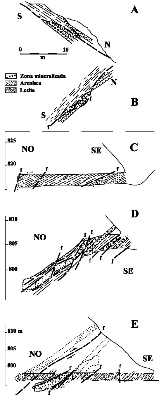
Fif Figura 14. Secciones geológicas de la mineralización de mercurio. Las ubicaciones aparecen en las figuras 6 y 7. Simplificado de LÓPEZ & BRINEMAN (1943).
