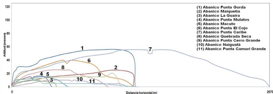
Gráfico 9. Perfiles topográficos transversales de los abanicos aluviales de la vertiente norte del macizo El Ávila, estado Vargas, Venezuela. Perfiles elaborados a partir de planos topográficos a escala 1:5.000 por DCN, 1958, Caracas; y planos topográficos del “Proyecto BITUCOTEX” a escala 1:5.000 por GDF, 1984, Caracas.
