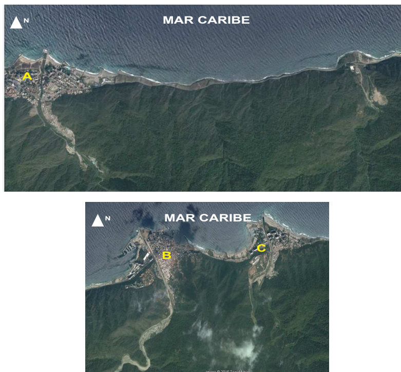
Gráfico 6. Vista aérea de los abanicos aluviales (A) Punta Cerro Grande, (B) Nai-guatá y (C) Punta Camurí Grande, vertiente norte del macizo El Ávila, estado Vargas, Venezuela. Imagen de satélite tomada de CNES/Astrium y Digital Globe por Google Earth, 2015.
