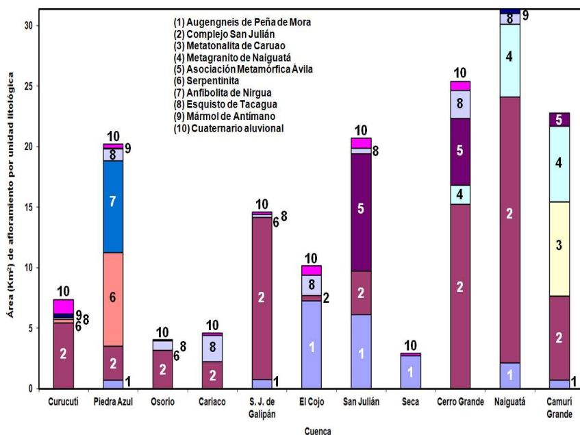
Gráfico 10. Áreas de afloramientos por unidades litológicas en cuencas de drenaje de la vertiente norte del macizo El Ávila, estado Vargas, Venezuela.
