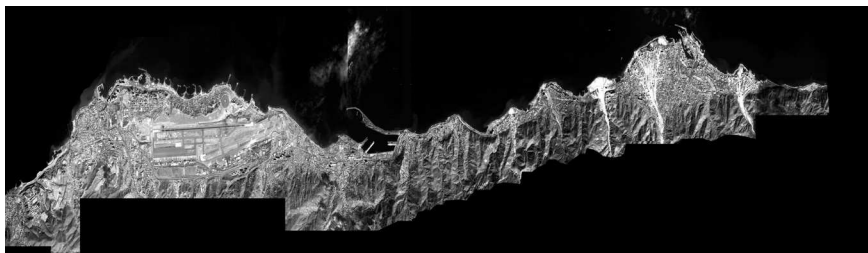
Gráfico 1. Imagen en la que destacan en color blanco y con mayor reflectancia, los depósitos del evento de aludes torrenciales de Diciembre de 1999 ocurridos en la vertiente norte del macizo El Ávila (estado Vargas, Venezuela), sobre los abanicos aluviales (de izquierda a derecha) Macuto, Punta El Cojo, Camurí Chiquito, Punta Caribe y Punta Cerro Grande. Imagen pancromática tomada del satélite “IKONOS” con resolución espacial de 1 metro por píxel por Centro de Procesamiento Digital de Imágenes [CPDI], 1999, Baruta.
